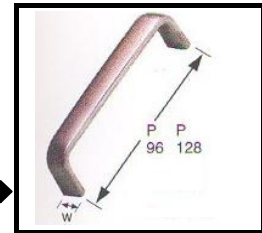
A-333 SUS OVAL DRAWER PULL
