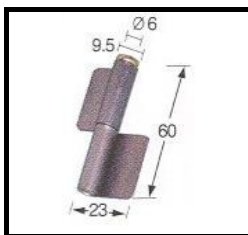
60# -1 MILD STEEL DOOR HINGE
