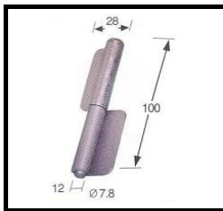
100# -1 MILD STEEL DOOR HINGE
