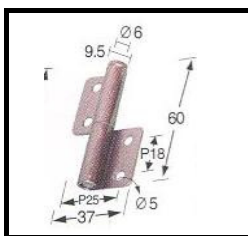
60# -1-4 MILD STEEL DOOR HINGE
