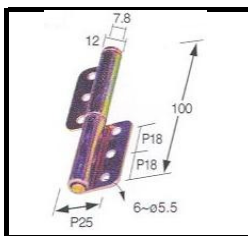
100# -1-4 MILD STEEL DOOR HINGE
